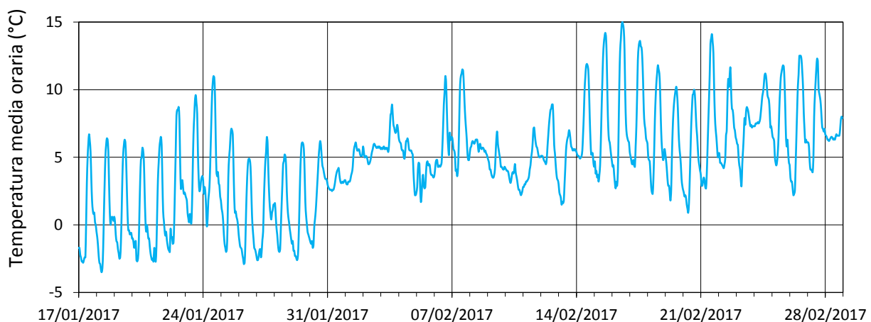
Figure 8: Temperatura dell'aria (media oraria).
