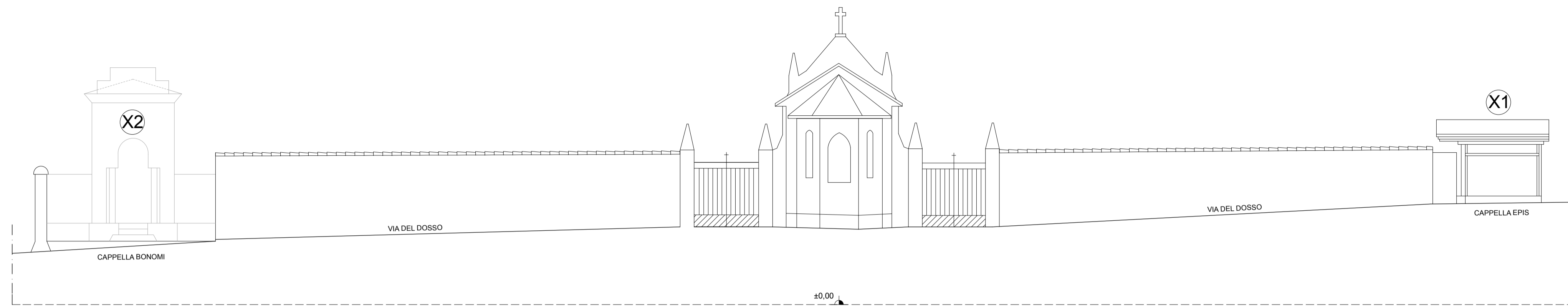
PROSPETTO DA VIA DEL DOSSO
